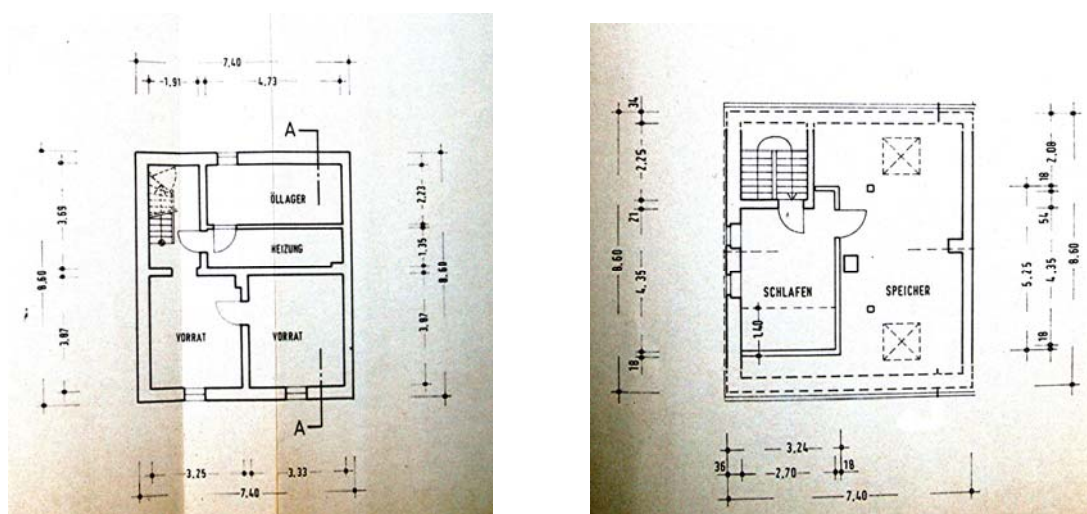
Bild 33: Haus Mertens, Kellergeschoss (links), Dachgeschoss (rechts) 56
