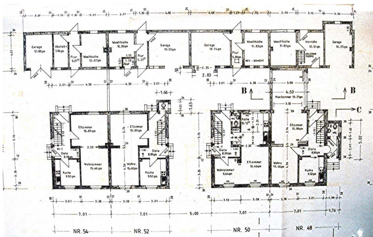
Bild 23: Gebäudegrundrisse Erdgeschoss der Häuser Nr. 48 (ganz rechts), 50, 52 und 54 (ganz links) 45
