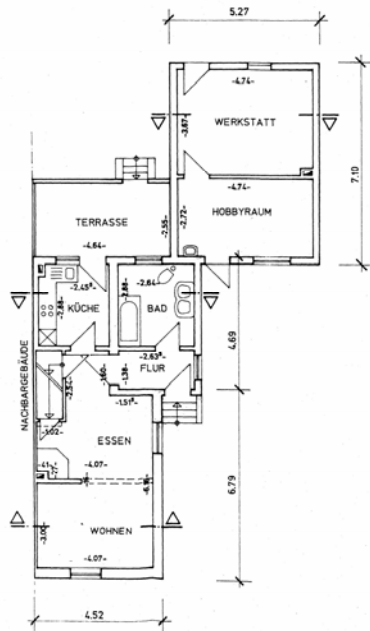
Bild 47: Haus Gesoleistraße Nr.2 (Baujahr 1936/1937); [links Grundriss Erdgeschoss]
