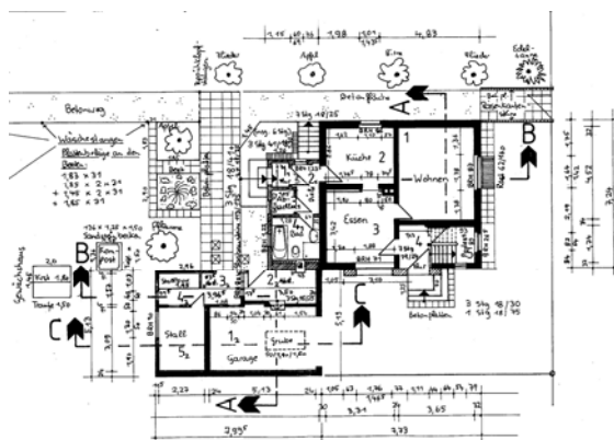
Bild 50: Haus Auf der Heide Nr.3 (Baujahr 1949); [links Grundriss Erdgeschoss]
