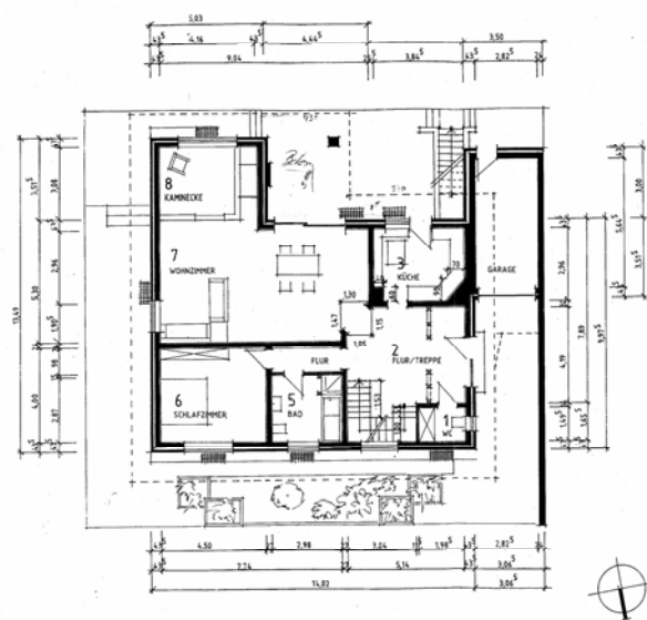
Bild 55: Haus Im Schaalendorf Nr.4 (Baujahr 1987); [unten Grundriss Erdgeschoss]
