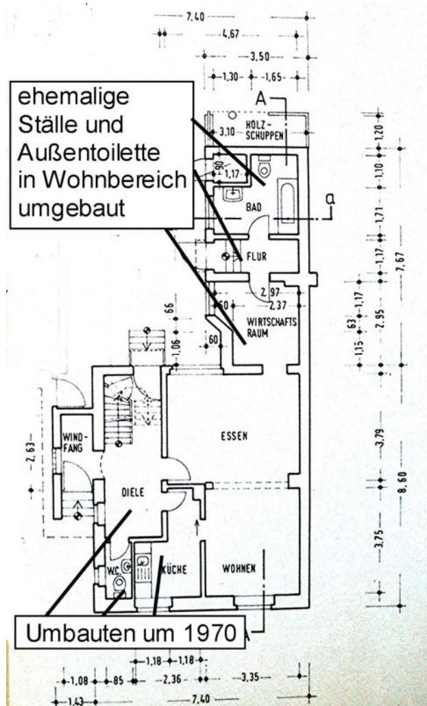
Bild 31: Haus Mertens, Erdgeschoss
