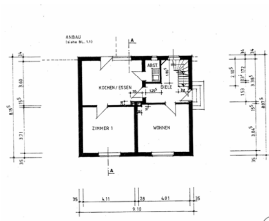
Bild 49: Haus Auf der Heide Nr.1 (Baujahr 1950); [links Grundriss Erdgeschoss]
