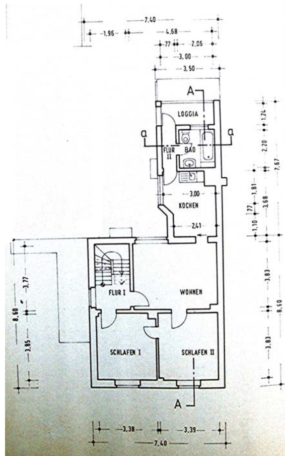
Bild 32: Haus Mertens, Obergeschoss
