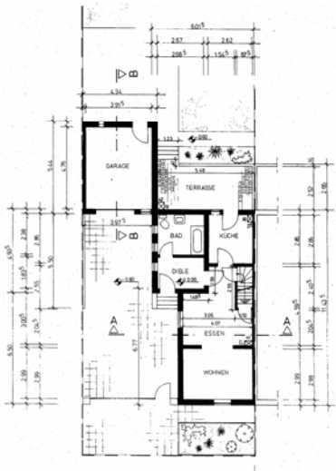
Bild 48: Haus Gesoleistraße Nr. 4 (Baujahr 1936/1937); [links Grundriss Erdgeschoss]
