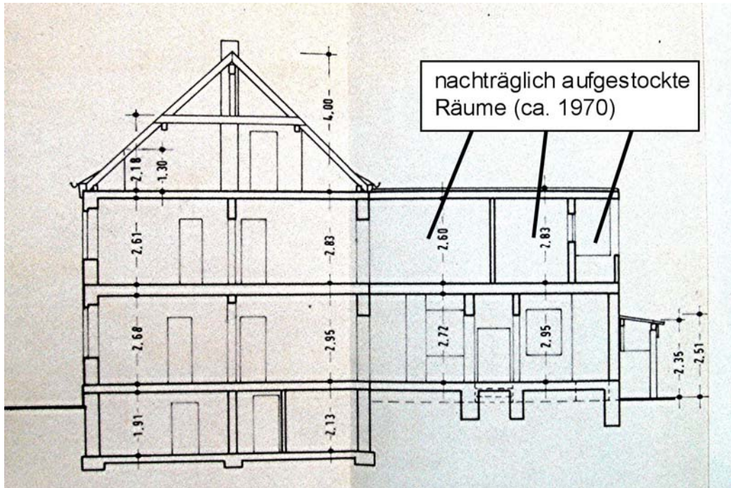
Bild 30: Schnitt durch das Haus Mertens
