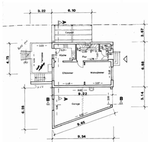
Bild 53: Haus Zur Rauhen Eiche Nr.7 (Baujahr 1965); [links Grundriss Erdgeschoss]
